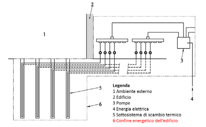
Figura 11.12 Sottosistema di estrazione geotermico con scambiatori verticali.
