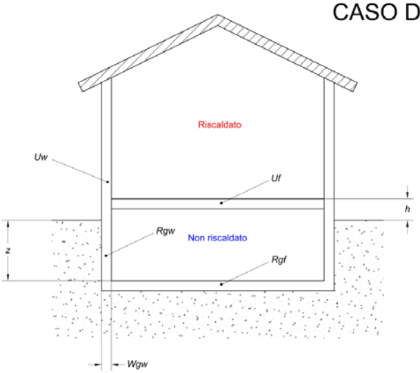
Figura B. 8 – Basamento CASO D - Piano interrato non climatizzato
