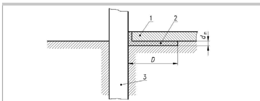
Figura B. 2 - Isolamento perimetrale orizzontale
