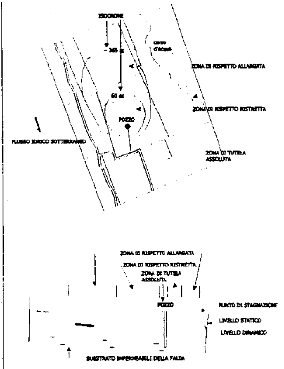
Figura 1 - esemplificazione della delimitazione delle aree di salvaguardia di un pozzo
