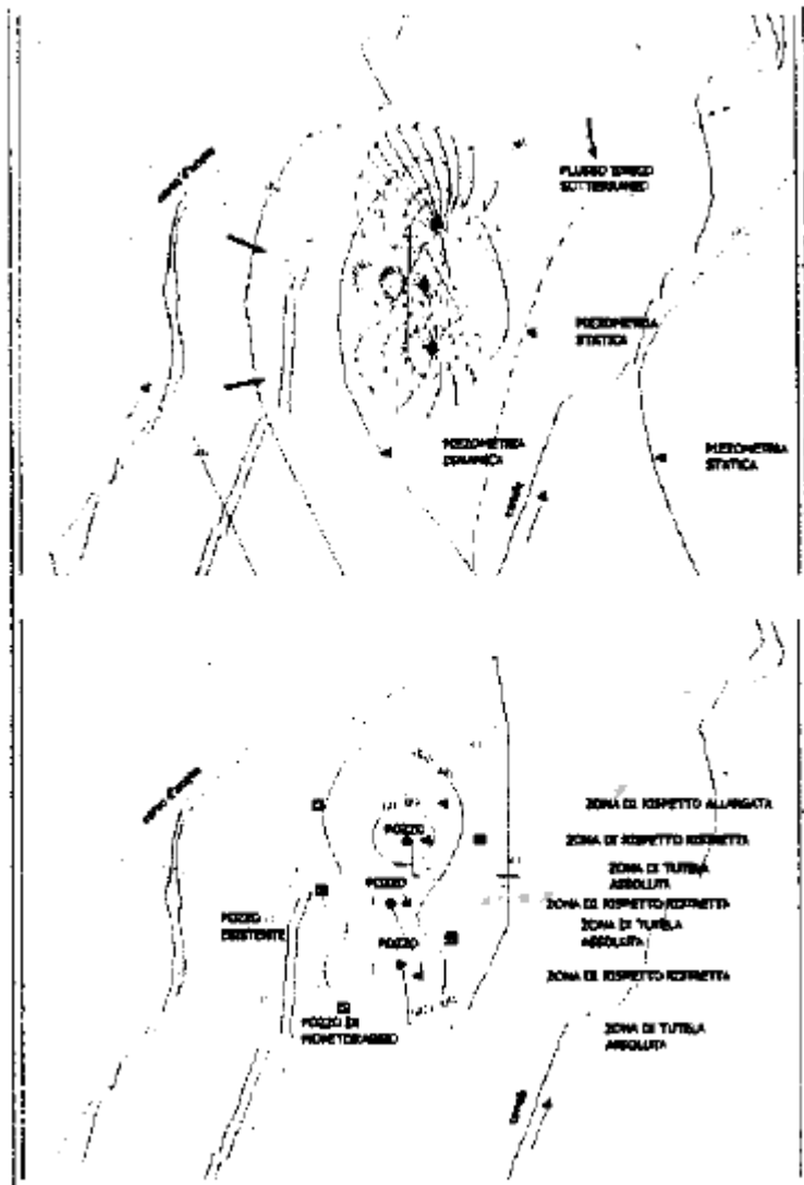
Figura 2 - Esempificazione della delimitazione delle aree di salvaguardia di piu' pozzi
